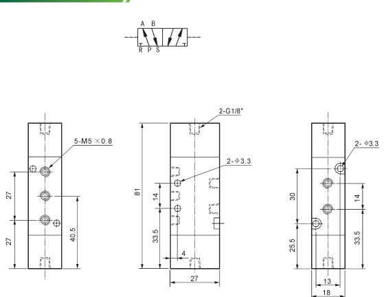
4A120-M5
