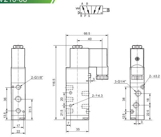
4V210-08
