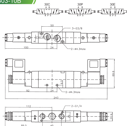
XG5303-10B
