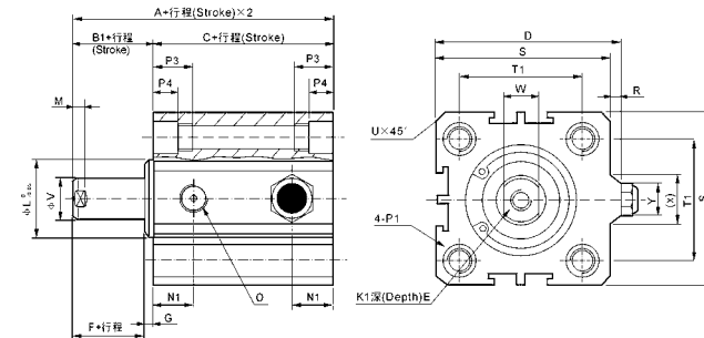
STA20-40
