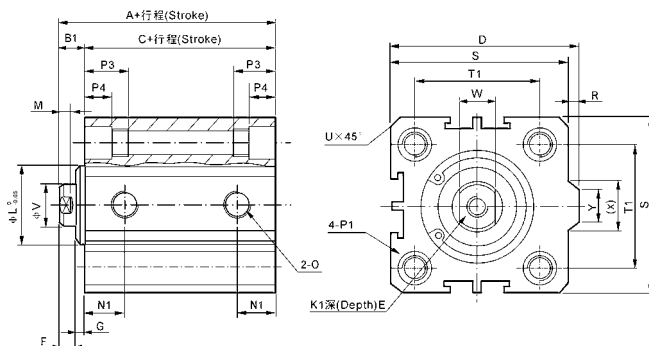
SDA20-100
