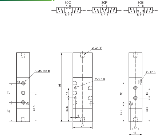
4A130-M5
