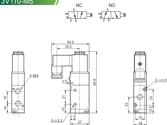
3V110-M5
